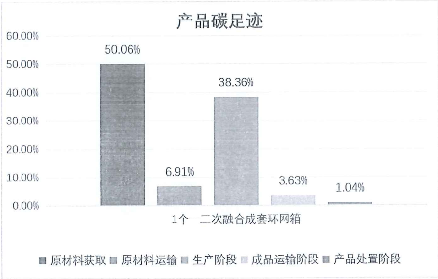
图 5.2-2 1 台一二次融合成套环网箱 产品生命周期阶段碳排放分布图
