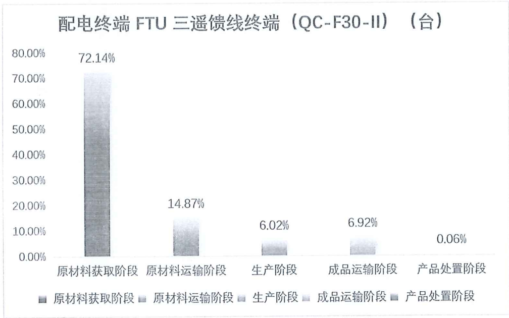
图 5.2-2 1 台配电终端 FTU 三遥馈线终端（QC-F30-II） 产品生命周期阶段碳排放分布图
