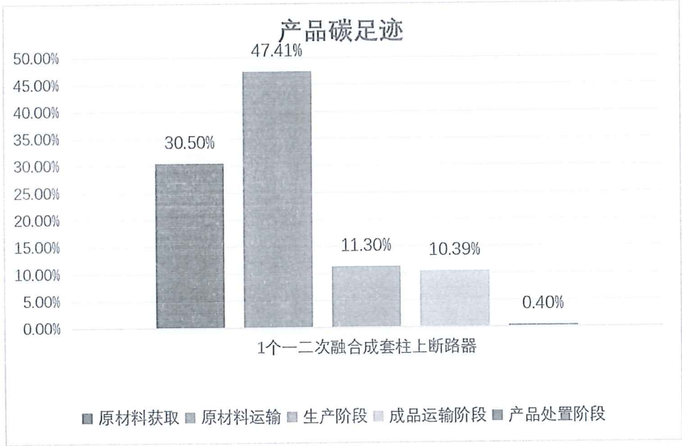
图 5.2-2 1 台一二次融合成套柱上断路器（ZW□-12/630-25、QC-F30-II） 产品生命周期阶段碳排放分布图
