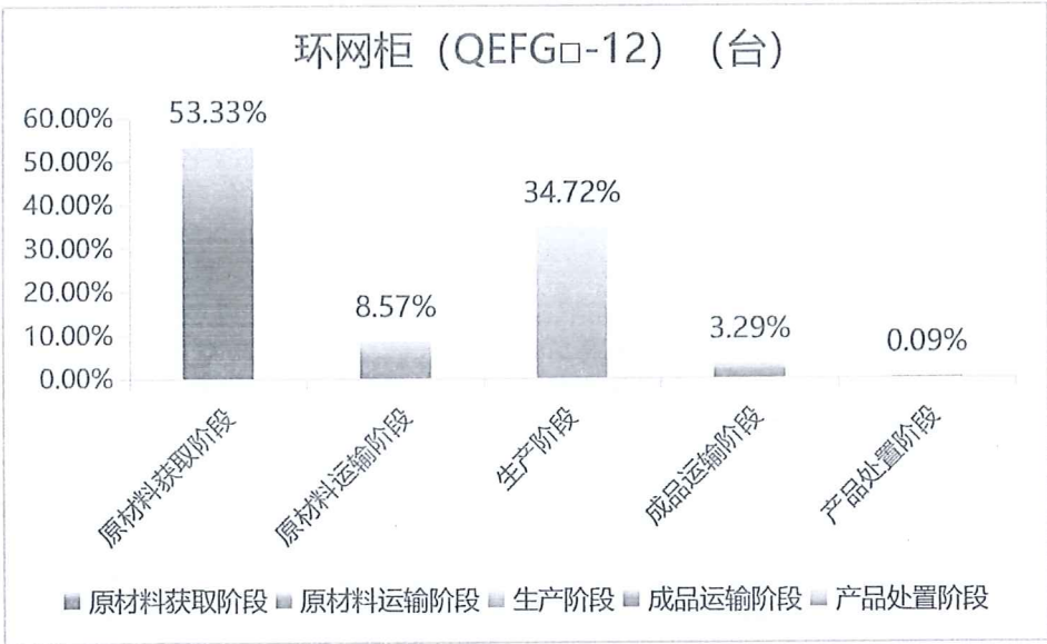
图 5.2-2 1 台环网箱（QEFW□-12） 产品生命周期阶段碳排放分布图
