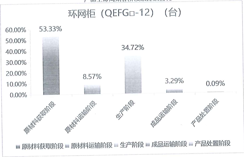
图 5.2-2 1 台环网柜（QEFG□-12） 产品生命周期阶段碳排放分布图
