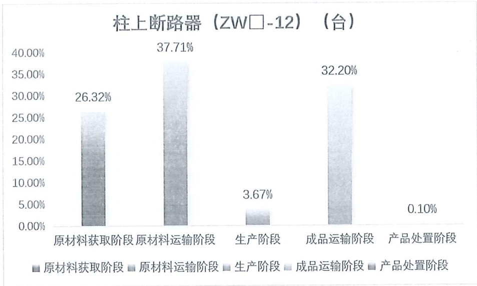
图 5.2-2 1 台柱上断路器（ZW□-12） 产品生命周期阶段碳排放分布图
