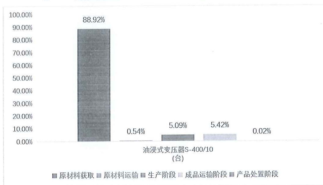
图 5.2-2 油浸式变压器（S-400/10） 生命周期阶段碳排放分布图
