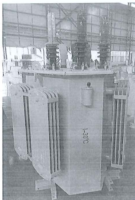
油浸式变压器 (S-400/10)
