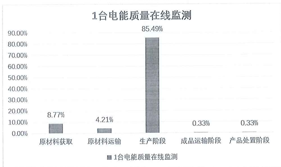
图 5.2-2 1 台电能质量在线监测（WR-108） 产品生命周期阶段碳排放分布图
