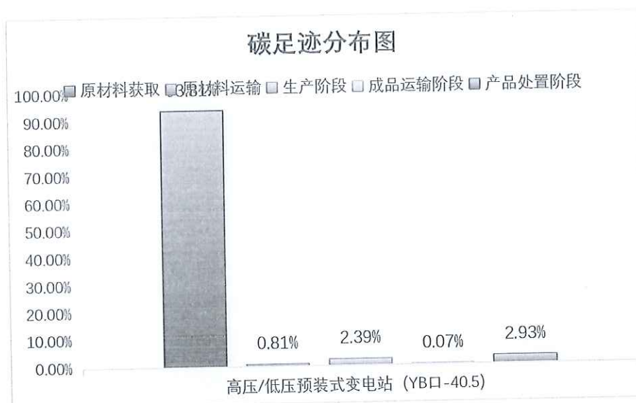
图 5.2.1-2 高压/低压预装式变电站（YB 口-40.5）产品生命周期阶段碳排放分布图
