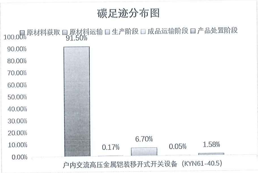
图 5.2.1-2 户内交流高压金属铠装移开式开关设备（KYN61-40.5）产品生命周期阶段碳排放分布图
