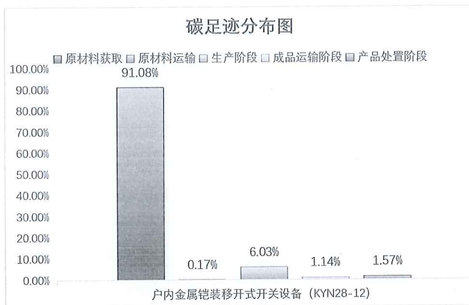
图 5.2.1-2 户内金属铠装移开式开关设备（KYN28-12）产品生命周期阶段碳排放分布图
