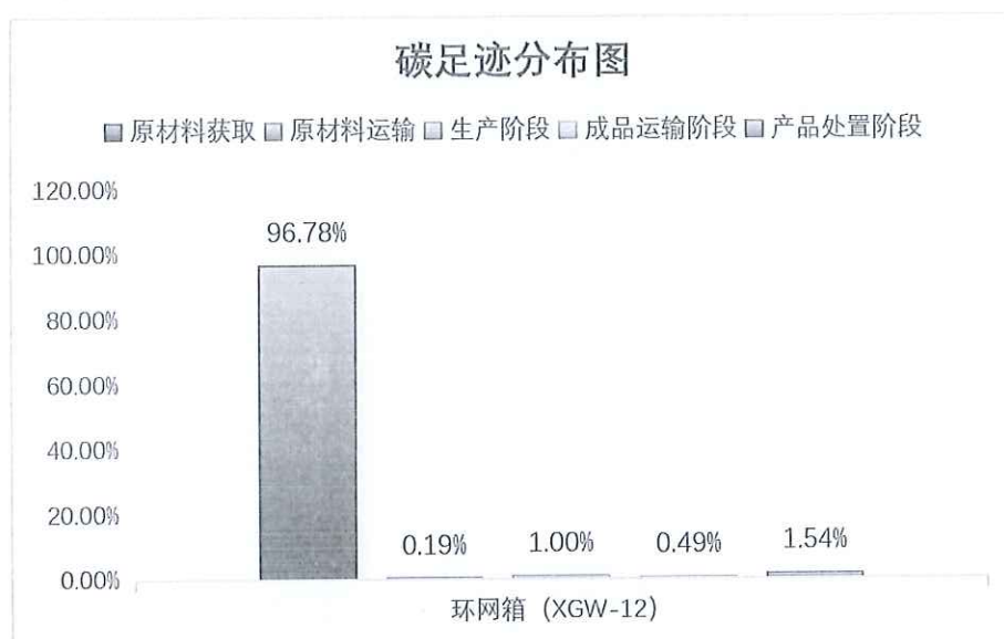
图 5.2.1-2 环网箱（XGW-12）产品生命周期阶段碳排放分布图
