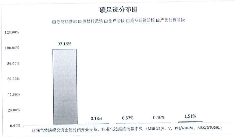
图 5.2.1-2 环保气体绝缘交流金属封闭开关设备、标准化站所终端集中式（MSE-12(V、V、PT)/630-20、MSK/DTU501）产品生命周期阶段碳排放分布图
