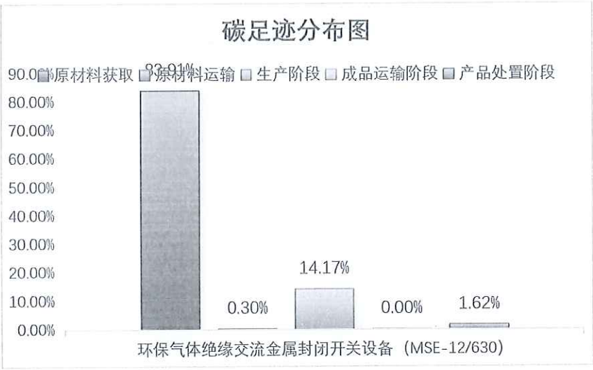
图 5.2.1-2 环保气体绝缘交流金属封闭开关设备（MSE-12/630）产品生命周期阶段碳排放分布图
