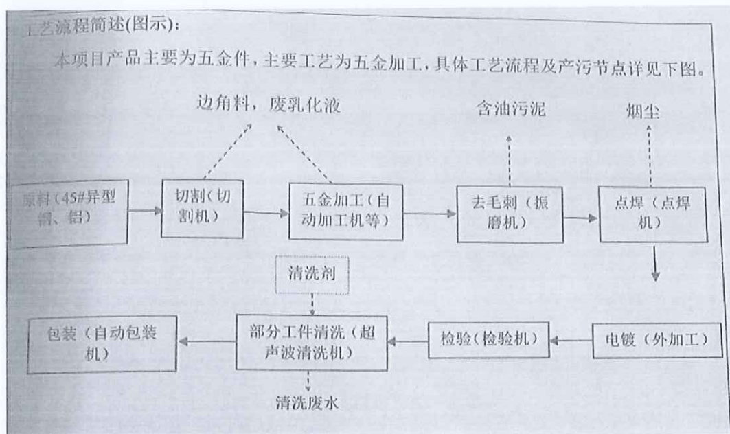
工艺流程图
