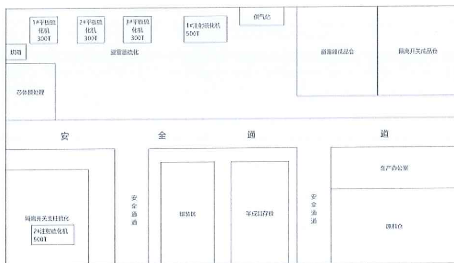
三#车间平面布置图
