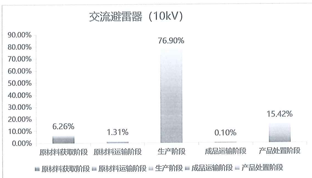
图 5.2-2 一只交流避雷器（10kV）生命周期阶段碳排放分布图
