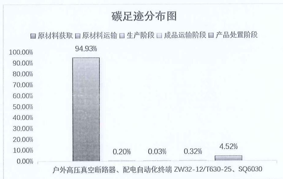
图 5.2.1-2 户外高压真空断路器、配电自动化终端（ZW32-12/T630-25、SQ6030）产品生命周期阶段碳排放分布图
