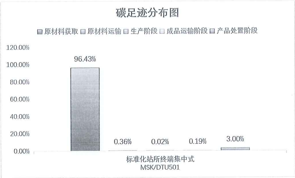
图 5.2.2-2 标准化站所终端集中式（MSK/DTU501）产品生命周期阶段碳排放分布图
