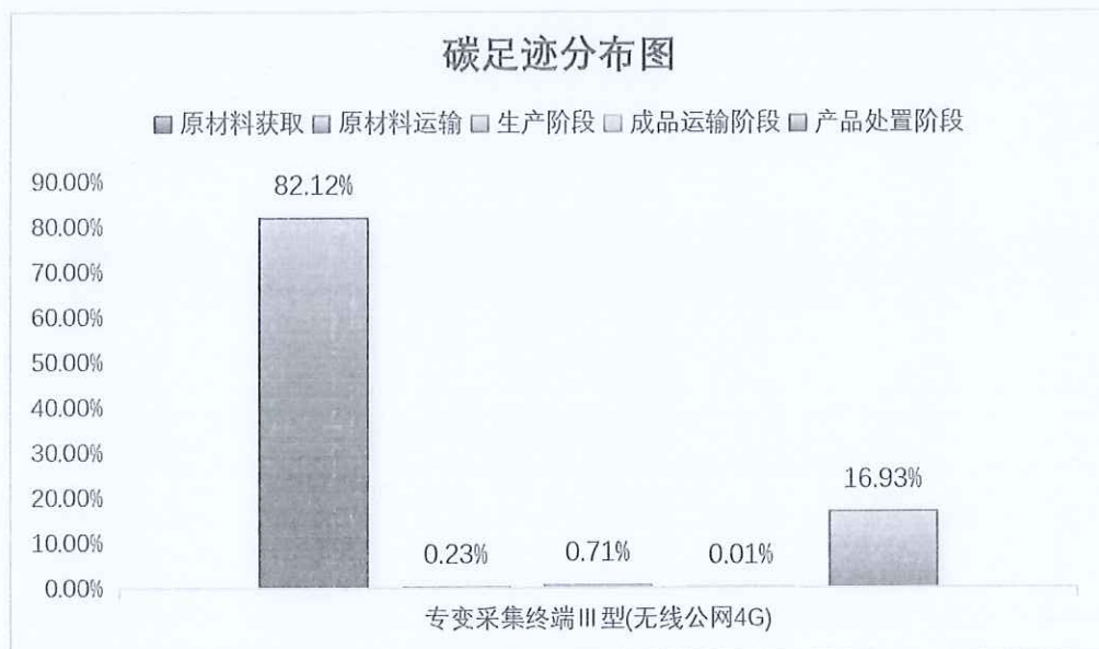
图 5.2.1-2 专变采集终端Ⅲ型(无线公网 4G)（FKTA43-MGCA05A）产品生命周期阶段碳排放分布图
