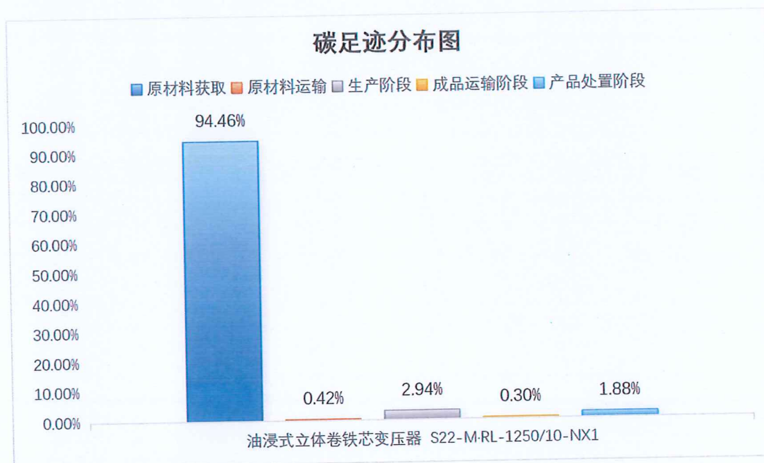
图 5.2.4-2 油浸式立体卷铁芯变压器（S22-M·RL-1250/10-NX1）产品生命周期阶段碳排放分布图
