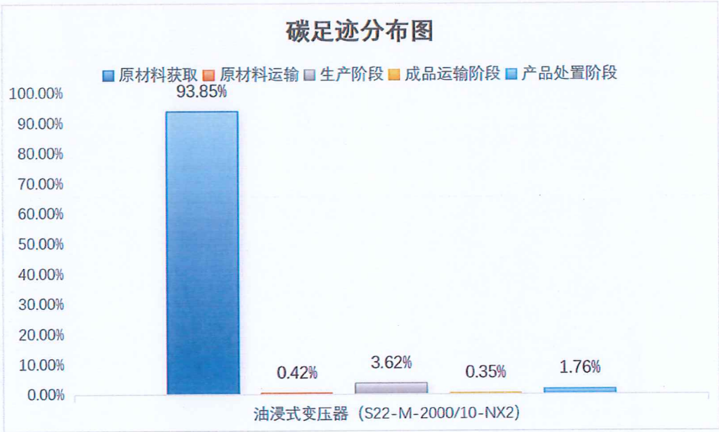
图 5.2.2-2 油浸式变压器（S22-M-2000/10-NX2）产品生命周期阶段碳排放分布图
