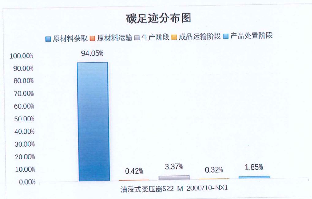
图 5.2.3-2 油浸式变压器（S22-M-2000/10-NX1）产品生命周期阶段碳排放分布图
