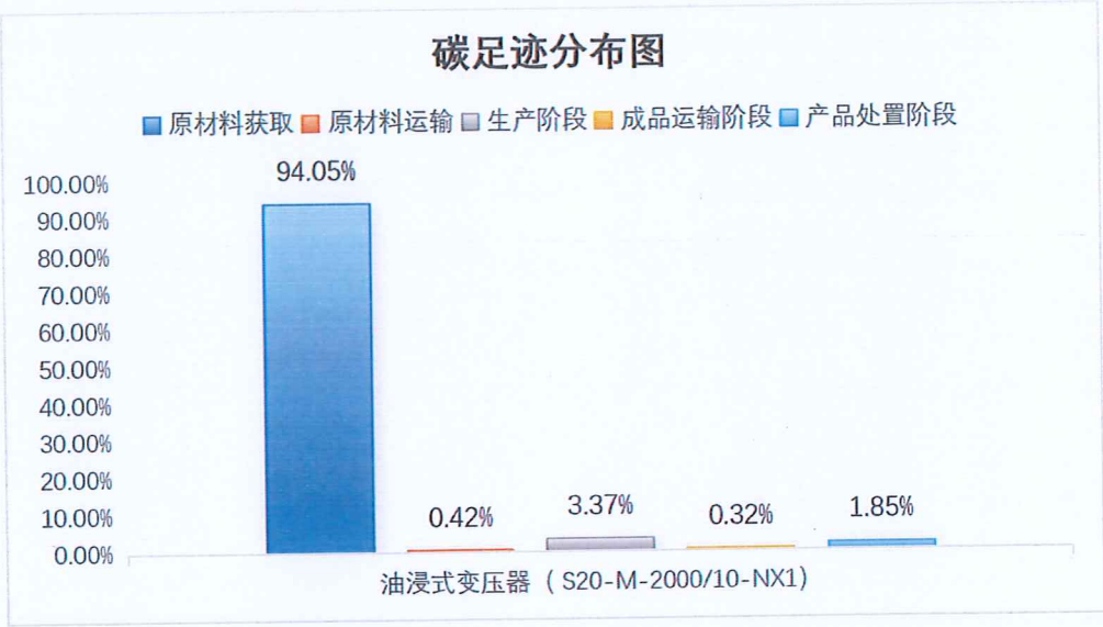
图 5.2.3-2 油浸式变压器（S20-M-2000/10-NX1）产品生命周期阶段碳排放分布图
