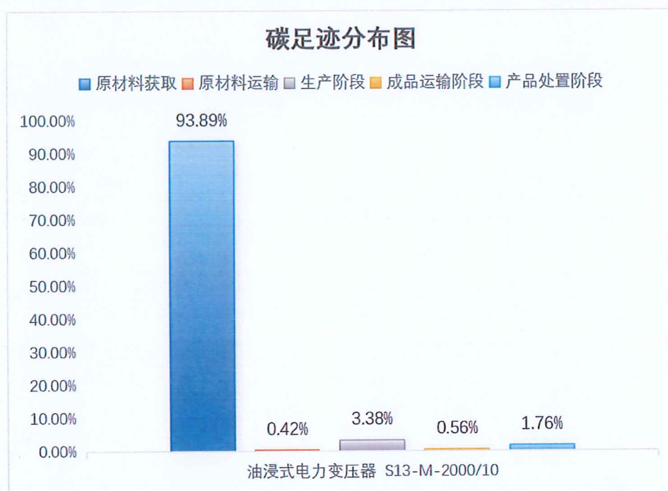
图 5.2.1-2 油浸式电力变压器（S13-M-2000/10）产品生命周期阶段碳排放分布图
