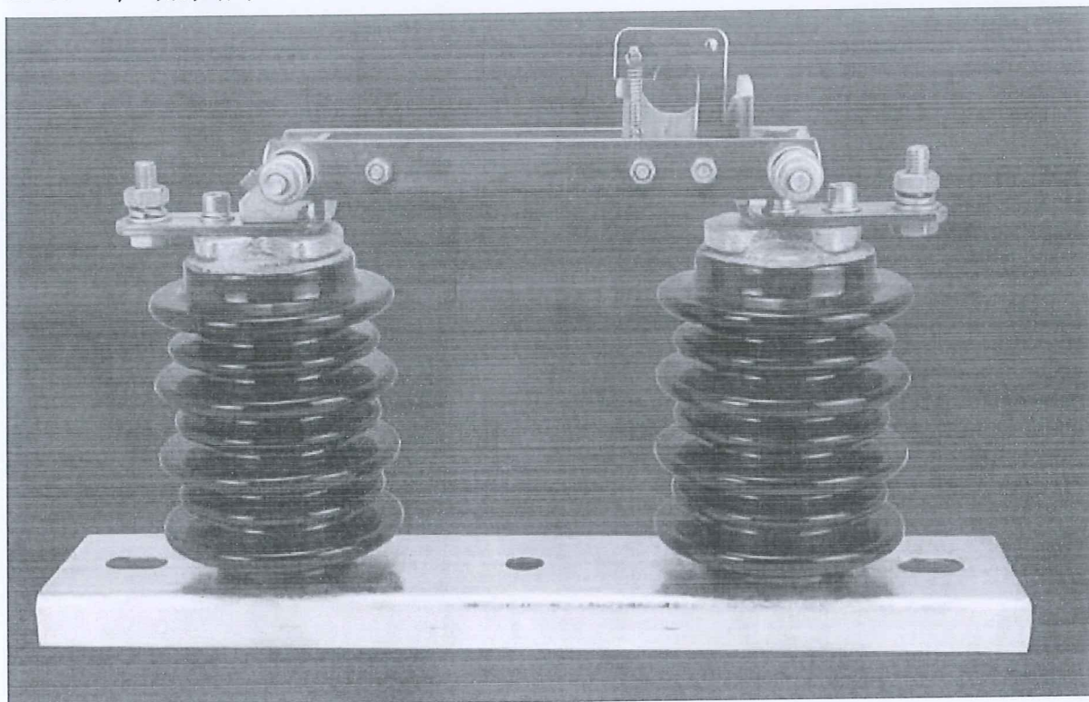
10KV 柱上隔离开关（复合材料）（HGW□-12/630-20）
