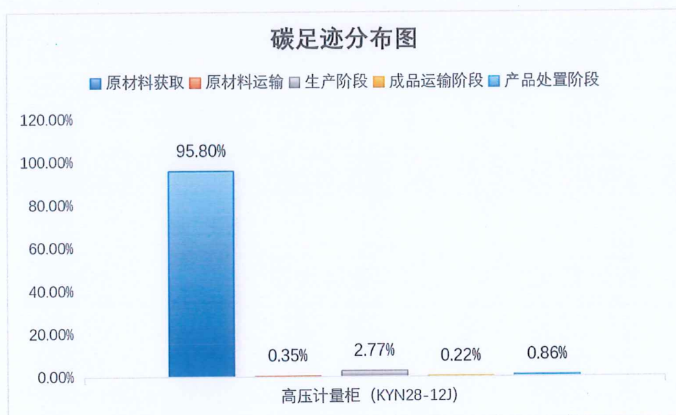
图 5.2-2 高压计量柜（KYN28-12J）产品生命周期阶段碳排放分布图
