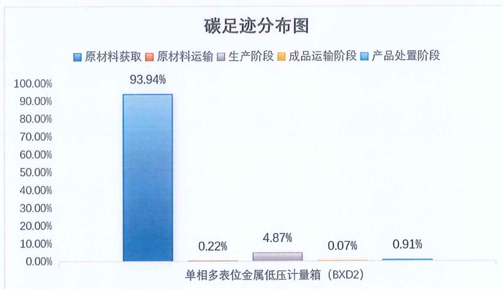
图 5.2-2 单相多表位金属低压计量箱（BXD2）产品生命周期阶段碳排放分布图
