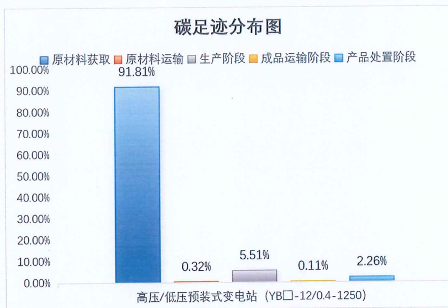
图 5.2-2 高压/低压预装式变电站（YB□-12/0.4-1250）产品生命周期阶段碳排放分布图
