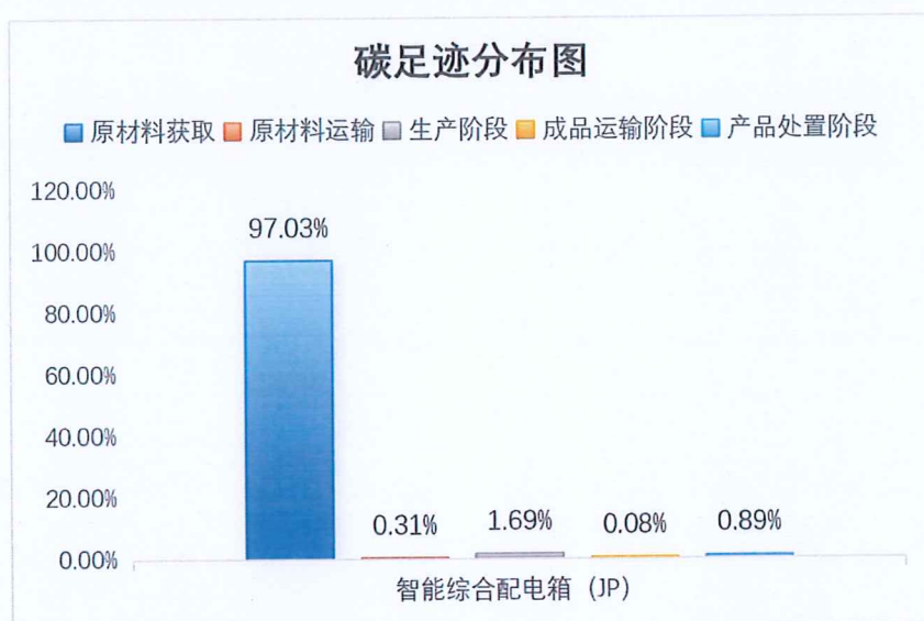
图 5.2-2 智能综合配电箱（JP）产品生命周期阶段碳排放分布图
