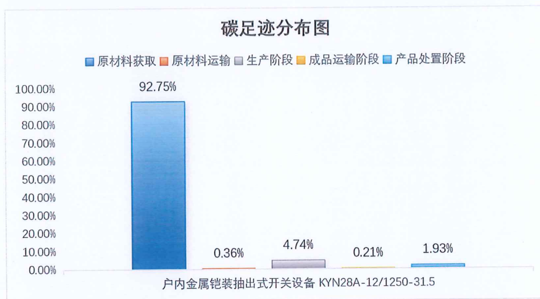
图 5.2-2 户内金属铠装抽出式开关设备 KYN28A-12/1250-31.5 产品生命周期阶段碳排放分布图
