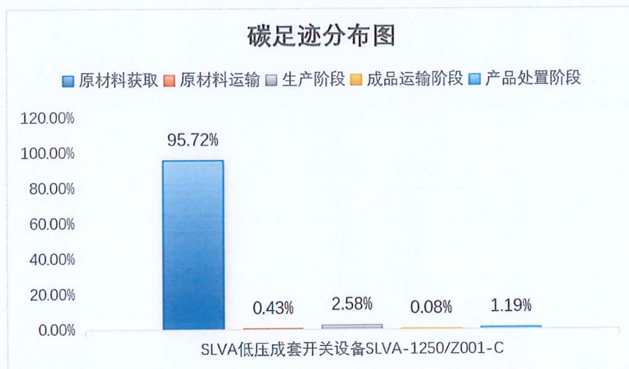
图 5.2-2 SLVA 低压成套开关设备 SLVA-1250/Z001-C 产品生命周期阶段碳排放分布图
