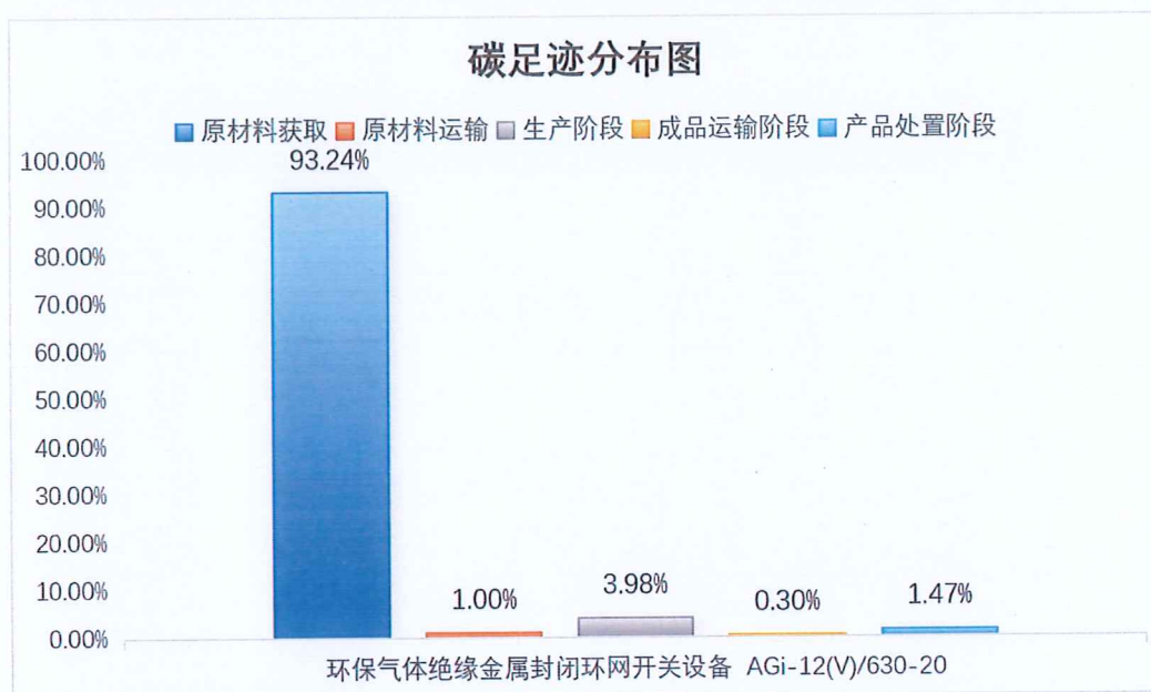
图 5.2-2 环保气体绝缘金属封闭环网开关设备 AGi-12(V)/630-20 产品生命周期阶段碳排放分布图
