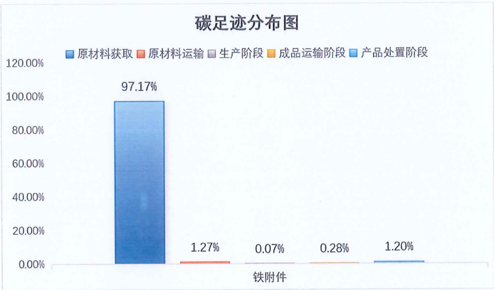
图 5.2.1-2 铁附件产品生命周期阶段碳排放分布图
