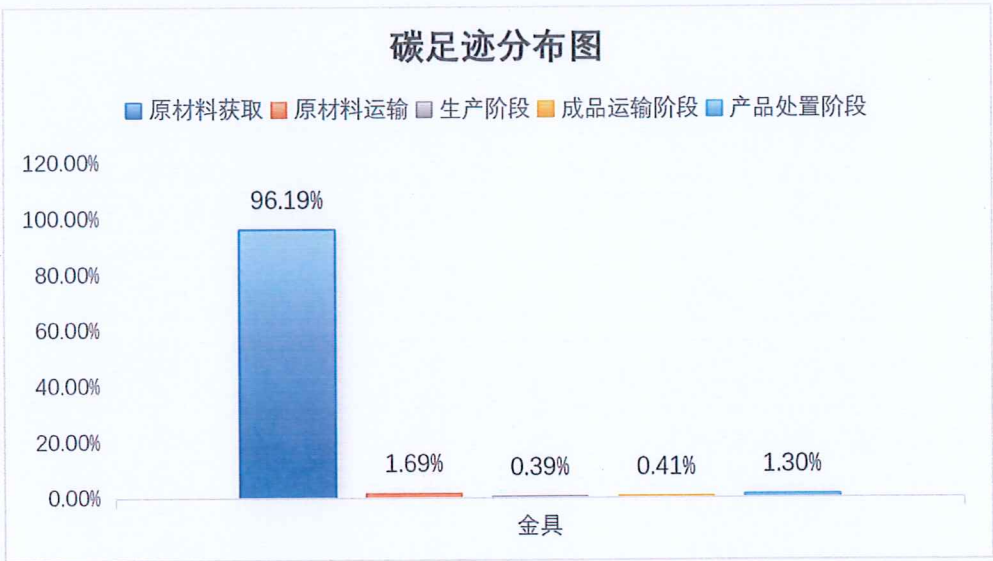
图 5.2.2-2 金具产品生命周期阶段碳排放分布图
