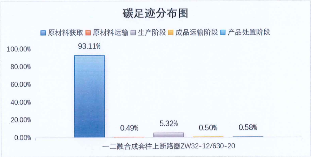
图 5.2-2 一二融合成套柱上断路器 ZW32-12/630-20 产品生命周期阶段碳排放分布图
