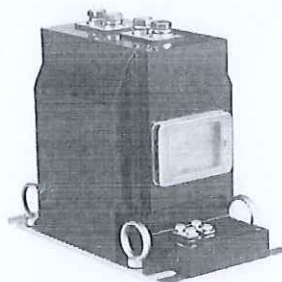
电流互感器（LJZN1-10）
