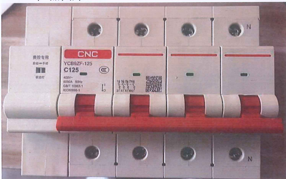
电能表外置断路器（小型重合闸）（YCB9ZF-125）
