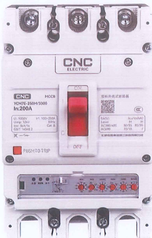
塑料外壳式断路器（电子式塑壳断路器）（YCM7E）
