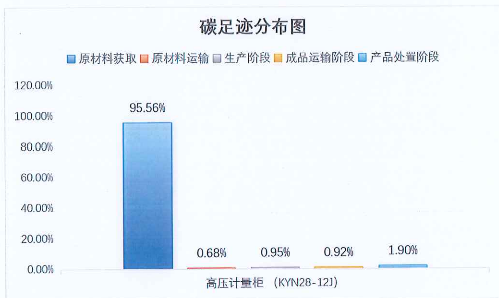
图 5.2-2 高压计量柜（KYN28-12J）生命周期阶段碳排放分布图
