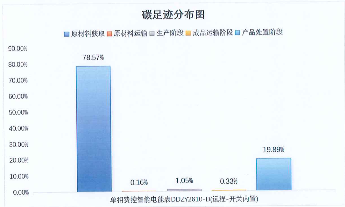
图 5.2.1-2 单相费控智能电能表 DDZY2610-D(远程-开关内置)生命周期阶段碳排放分布图
