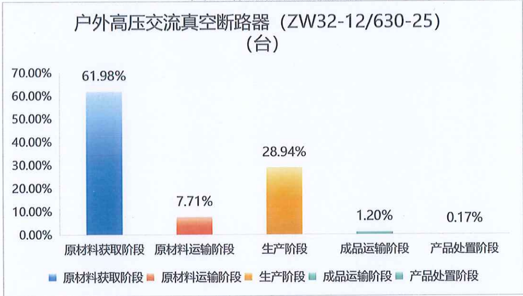
图 5.2-2 户外高压交流真空断路器（ZW32-12/630-25） 产品生命周期阶段碳排放分布图
