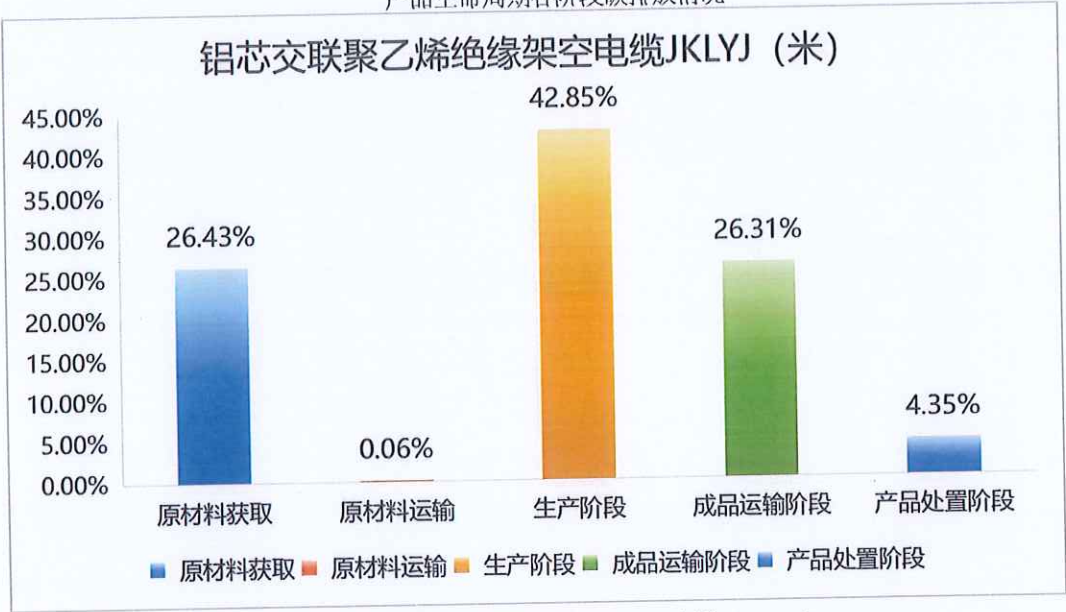
图 5.2-2 铝芯交联聚乙烯绝缘架空电缆（JKLYJ） 产品生命周期阶段碳排放分布图
