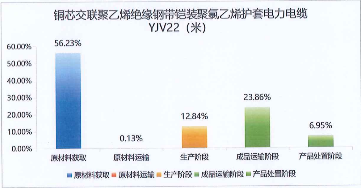
图 5.2-2 铜芯交联聚乙烯绝缘钢带铠装聚氯乙烯护套电力电缆（YJV22） 产品生命周期阶段碳排放分布图
