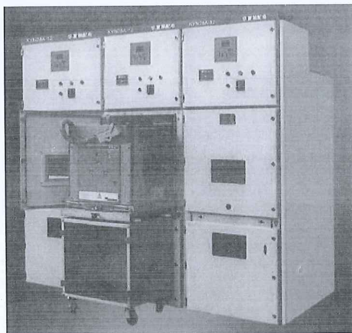
铠装移开式交流金属封闭开关设备（KYN28A-12）
