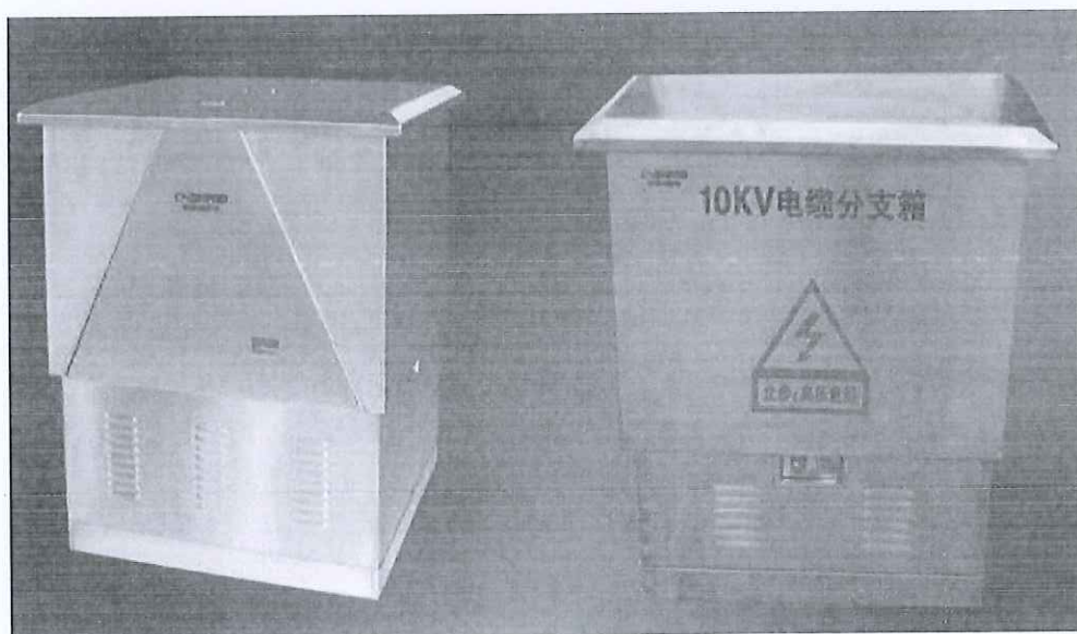
高压电缆分支箱 (DFW□-12)
