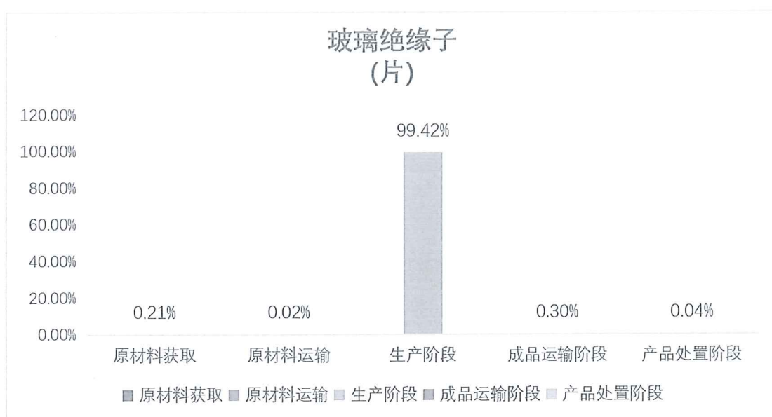
图 5.2.1-2 玻璃绝缘子（U70B）生命周期阶段碳排放分布图
