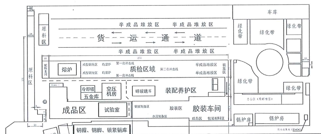
厂区平面图
