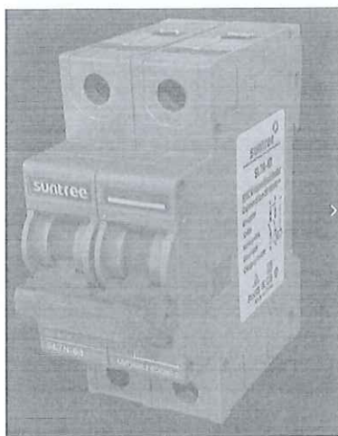
小型直流断路器 ( SL7N-63 4P 63A DC1000、1200V) DC1000、1200V)
