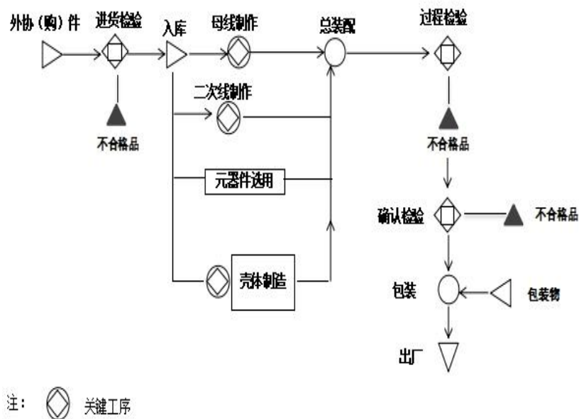
高压成套开关工艺流程图
