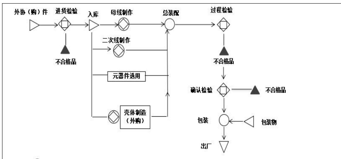
配电箱工艺流程图
