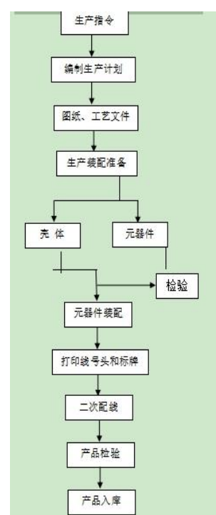
预装箱式变电站生产工艺流程图
