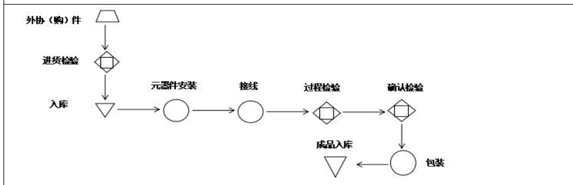
油浸式电力变压器工艺流程图
