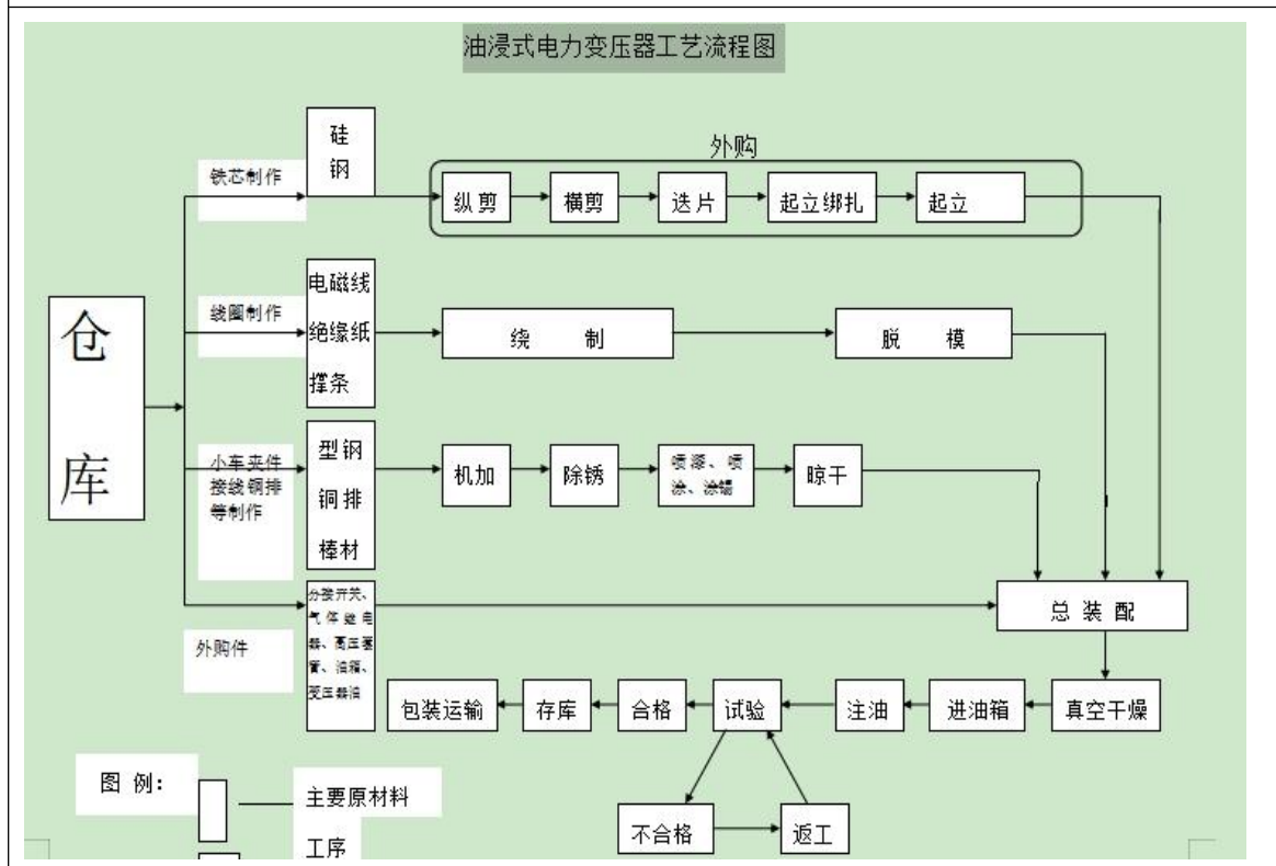
油浸式电力变压器工艺流程图
