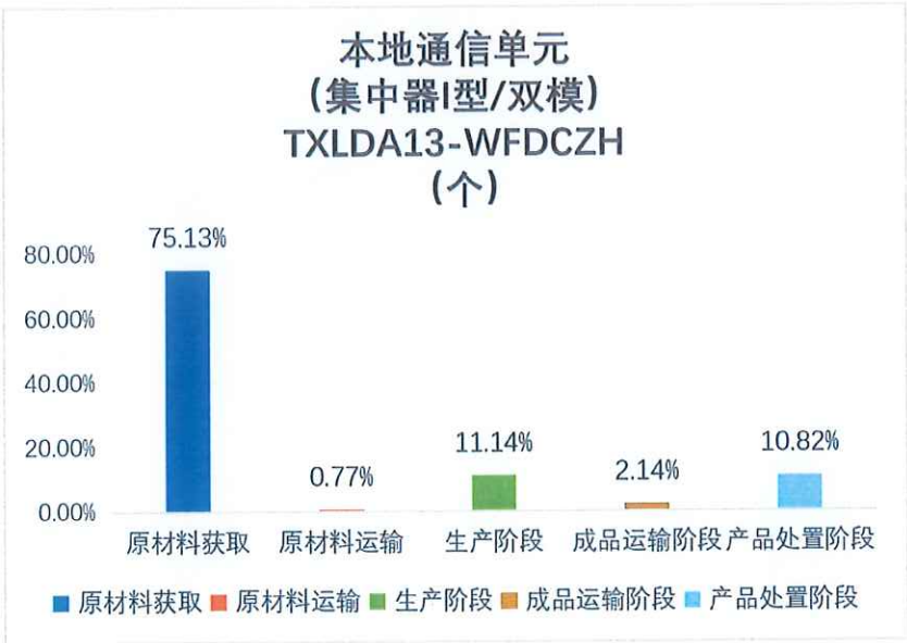
图 5.2-2 本地通信单元（集中器 I 型/双模） 生命周期阶段碳排放分布图
