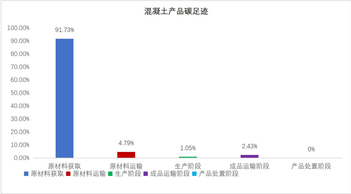
图 5.2-2 混凝土生命周期阶段碳排放分布图
