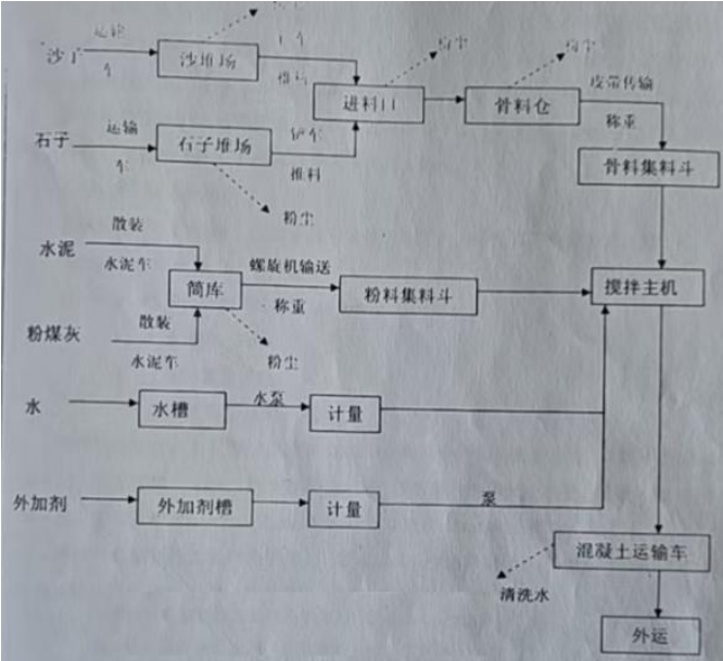
工艺流程图
