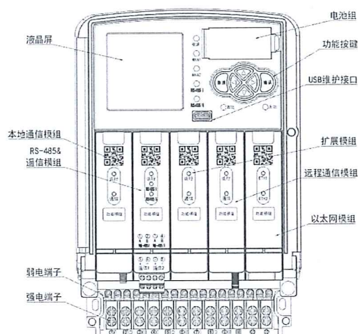
图 2.2 终端外观结构示意图
