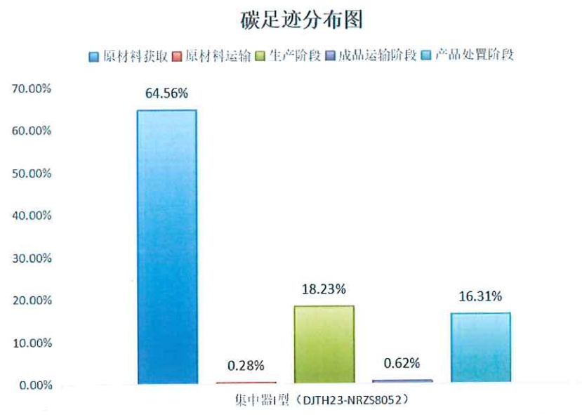
图 5.2-2 集中器 I 型（DJTH23-NRZS8052）生命周期阶段碳排放分布图
