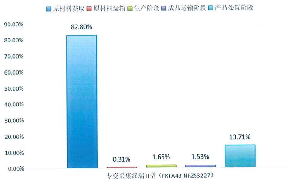
图 5.2-2 专变采集终端 III 型（FKTA43-NRZS3227） 生命周期阶段碳排放分布图
