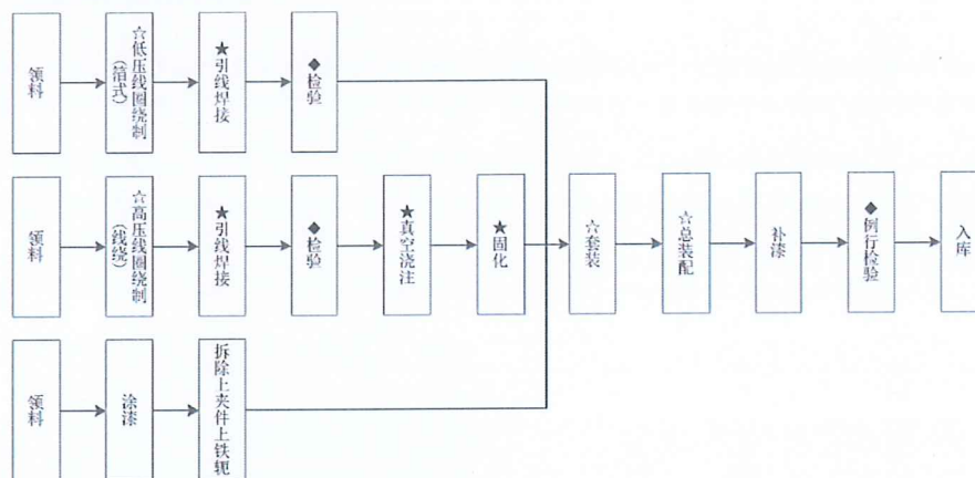
干式变压器实现过程流程图
