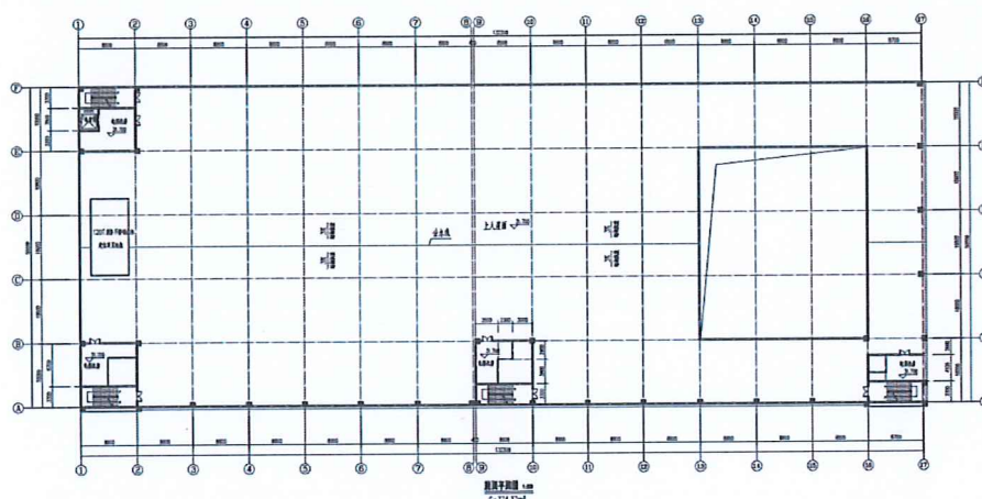
厂区布局图
