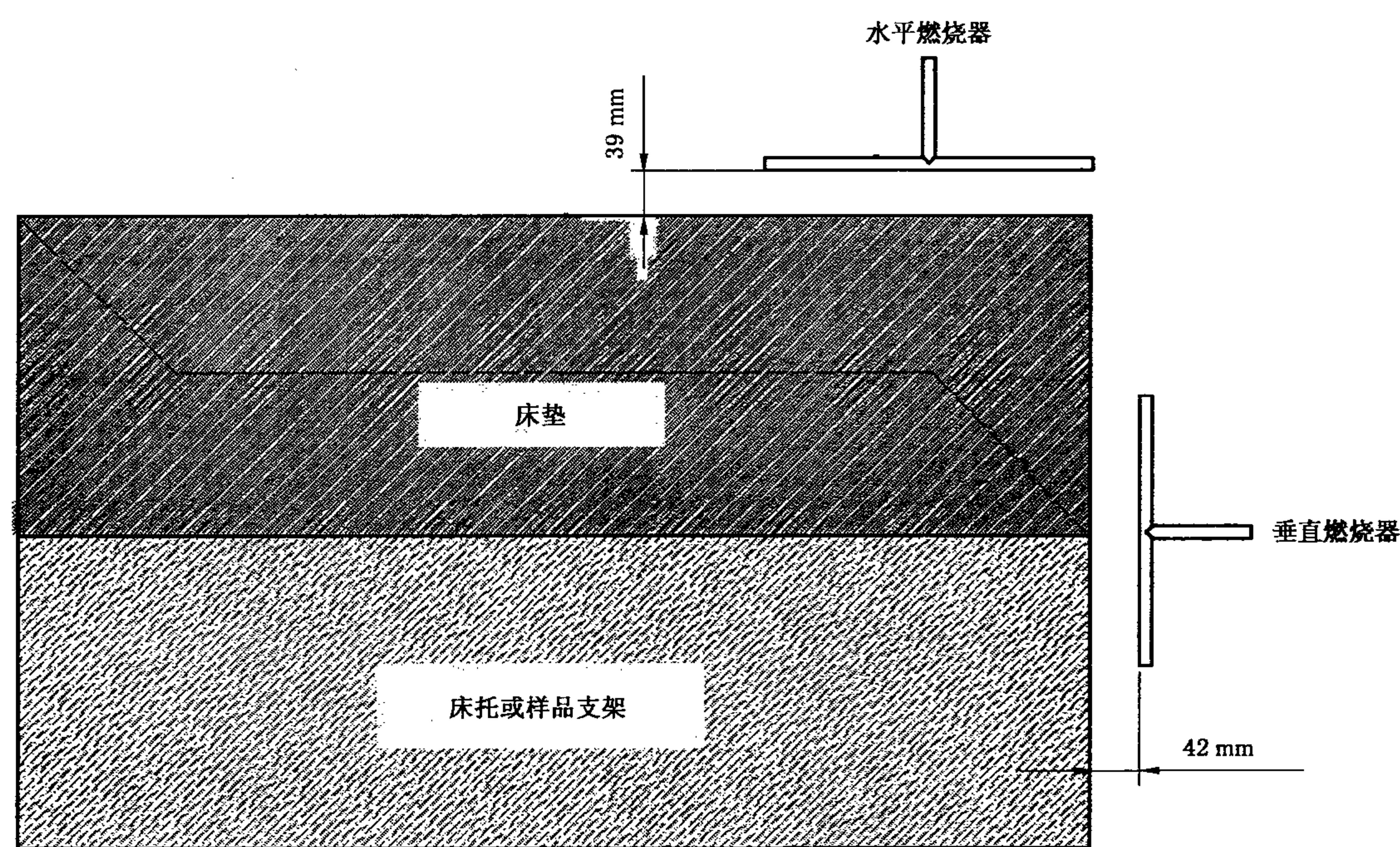
a) 侧视图
