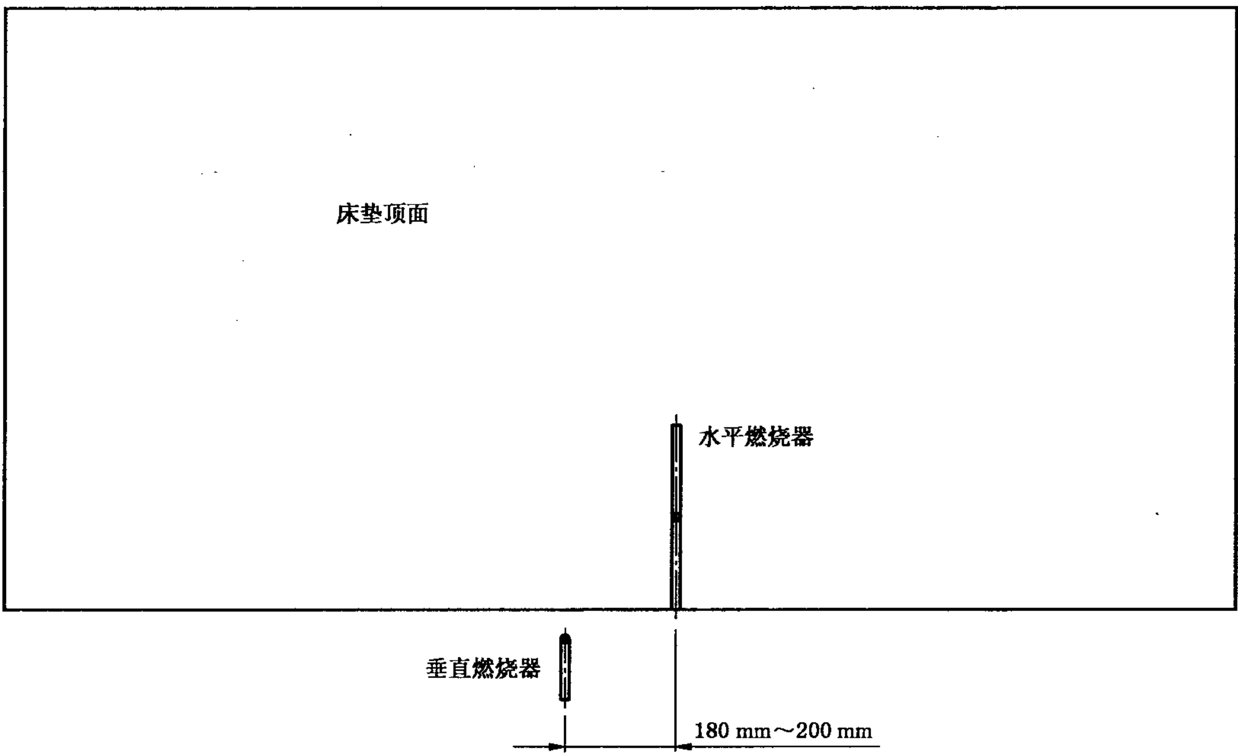
b) 俯视图
