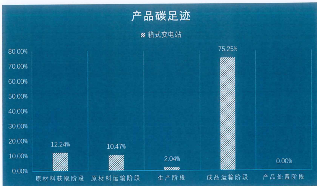
图 5.2-4.2 生命周期阶段碳排放分布图
