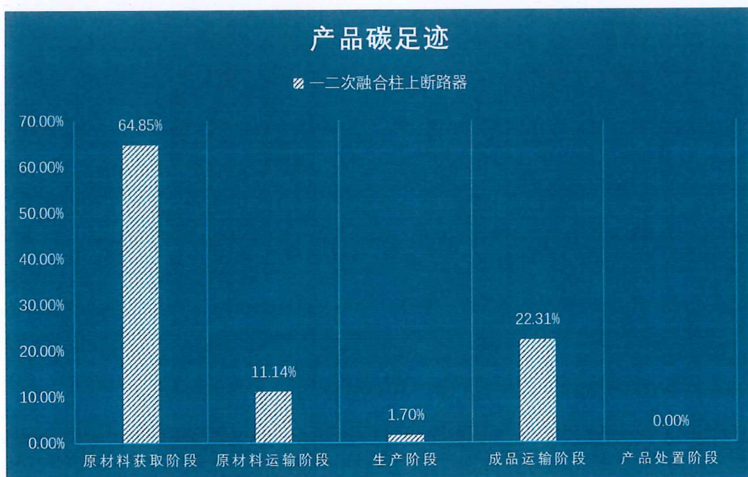
图 5.2-2.2 生命周期阶段碳排放分布图
