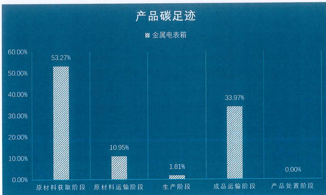
图 5.2-3.2 生命周期阶段碳排放分布图
