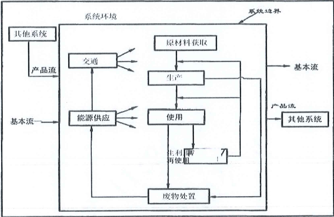
图 3.2: 产品系统边界示意图
