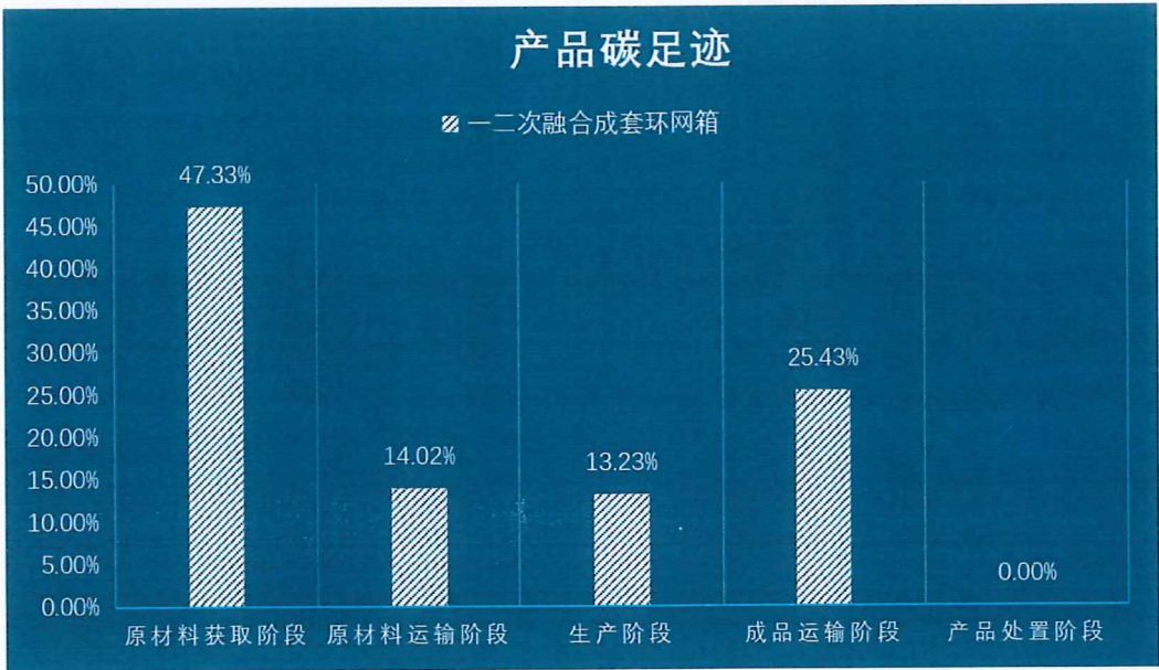
图 5.2-1.2 生命周期阶段碳排放分布图
